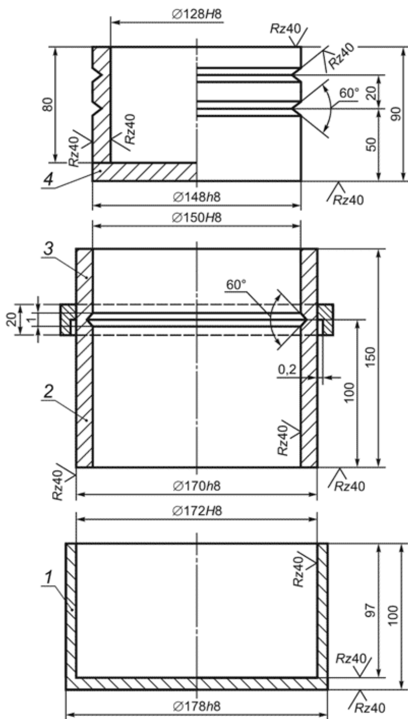
1 - поддон; 2 - цилиндр; 3 - приставка; 4 - пуансон
